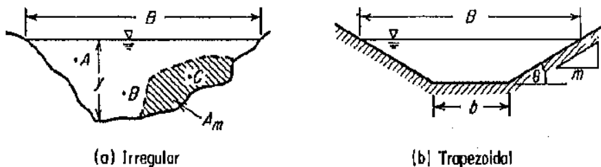
Figura 1 - Seção de Canal Irregular Típica e suas variáveis correspondentes para a consideração de um Canal Trapezoidal Regular.
